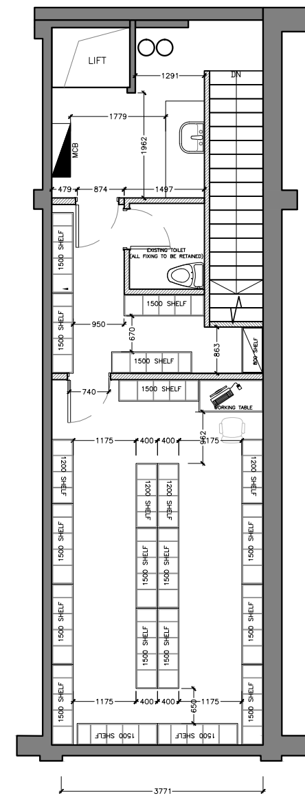
2F
