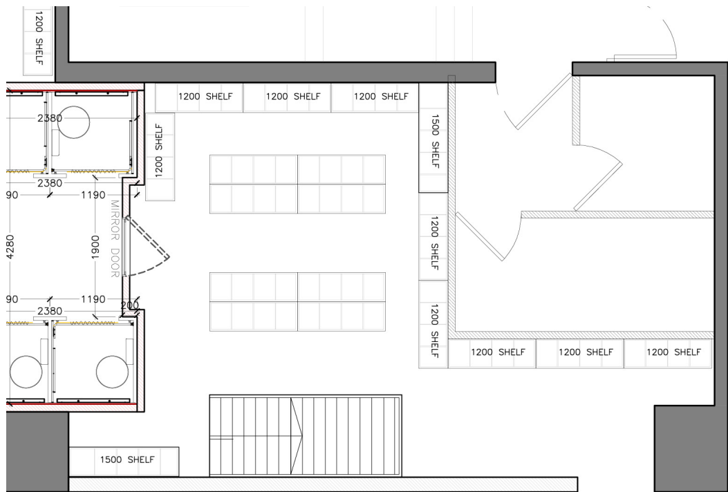
G/F
